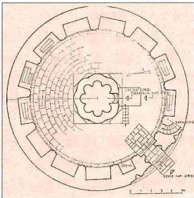
Mama Hatun Türbesi ve türbesinin planı - Tercan / Erzincan
